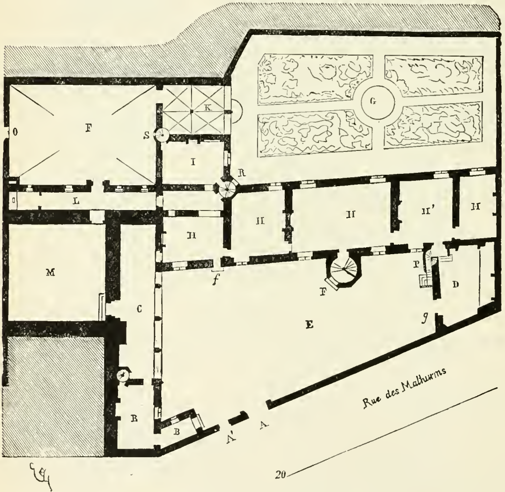
FIG. 183. Paris: Hôtel de Cluny. 1490 to 1520 A.D. Plan.
